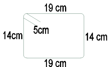
Εικόνα 7: Συνδετήρας για εγκάρσιο οπλισμό διαζώματος που τοποθετείται ανά 10 εκατοστά.
